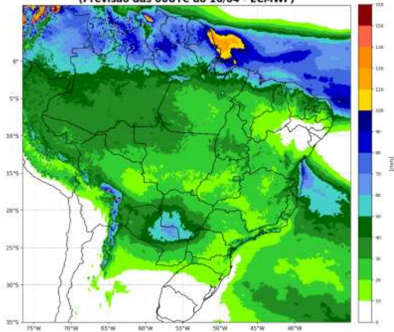
Precipitação acumulada (mm) entre os dias: 19/04 e 25/04 (semana 4) (Previsão das 00UTC do 16/04 - ECMWF)
