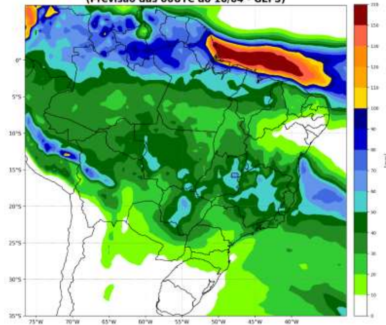
Precipitação acumulada (mm) entre os dias: 19/04 e 25/04 (semana 4) (Previsão das 00UTC do 16/04 - GEFS)
