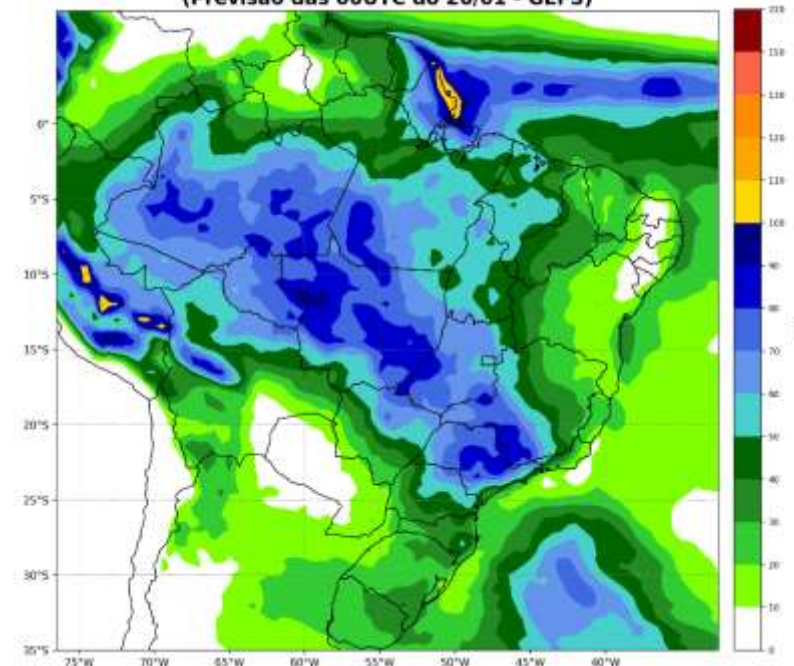
Precipitação acumulada (mm) entre os dias: 01/02 e 07/02 (semana 1) (Previsão das 00UTC do 26/01 - GEFS)
