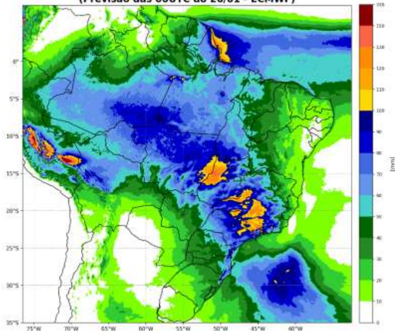
Precipitação acumulada (mm) entre os dias: 01/02 e 07/02 (semana 1) (Previsão das 00UTC do 26/01 - ECMWF)
