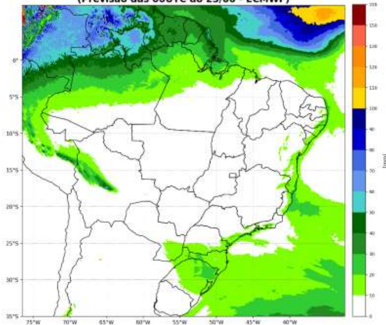
Precipitação acumulada (mm) entre os dias: 29/06 e 05/07 (semana 1) (Previsão das 00UTC do 25/06 - ECMWF)
