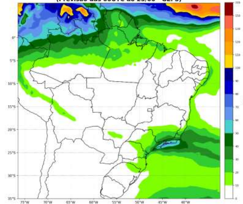
Precipitação acumulada (mm) entre os dias: 29/06 e 05/07 (semana 1) (Previsão das 00UTC do 25/06 - GEFS)
